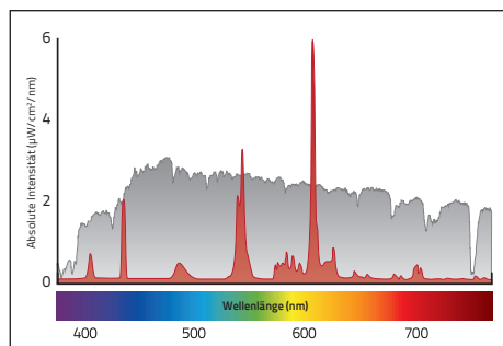
Typisches Lichtspektrum einer Energiesparlampe (Kompaktleuchtstofflampe)
