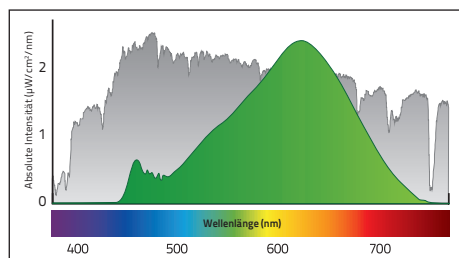
Das naturnahe Lichtspektrum der Pure-Z-Retro-LED
